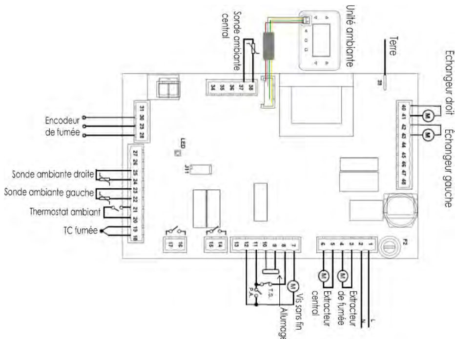
SCHEMA DE CONNEXION DE LA CARTE ÉLECTRONIQUE
